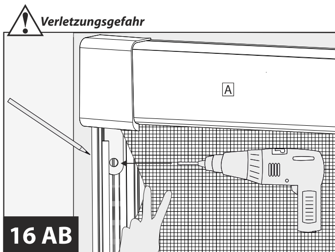
Insektenschutzgewebe etwas nach unten ziehen und gemäß Abb. 21 AB arretieren. Gewebe leicht nach hinten wegdrücken und seitliche Führungsprofile mit einem Ø 4 mm Metallbohrer vorbohren. Bohrloch auf das Mauerwerk übertragen. Wiederholen Sie diesen Vorgang auch für die gegenüberliegende Seite.
