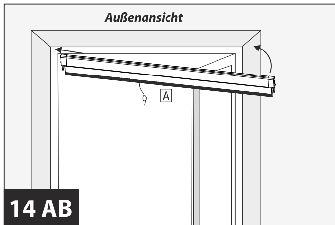
14 AB Rollokassette inkl. Griffleiste A in der Laibung verklebten!
