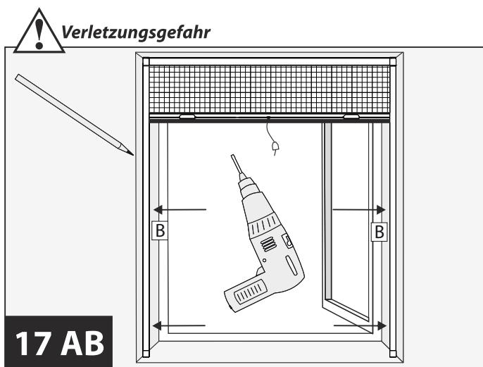
17 AB Seitliche Führungsprofile B jeweils gleichmäßig an zwei Stellen verteilt mit einem Ø 4 mm Metallbohrer vorbohren. Bohrlöcher auf das Mauerwerk übertragen.
