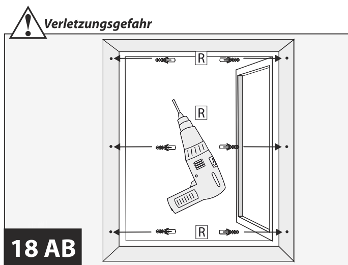
18 AB Rollobausatz wieder aus der Fensterlaibung herausnehmen. Mauerwerk an den markierten Positionen mit einem Ø 6 mm Steinbohrer vorbohren. Dübel R einsetzen. Achtung! Je nach Untergrund sind ggf. andere Schrauben, Dübel und Bohrer notwendig (Nicht im Lieferumfang enthalten).
